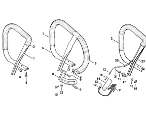
Trubka rukojeti, výhřevná fólie
