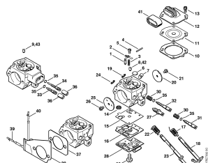
Karburátor HD-15, HD-17
