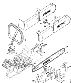
Přestavná sada "pila pro záchranné služby" (27.2000), (31.2005), (15.2007)
